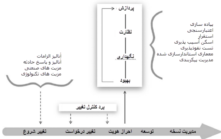
شکل 4.7. رابطه ی بین پردازش ها و مدیریت نسخه
